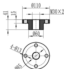
法兰端BP
