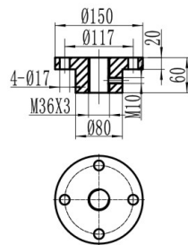
法兰端BP
