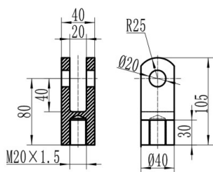
销孔端PO
