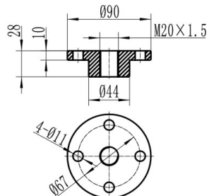
法兰端BP
